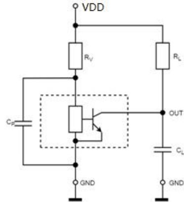
典型应用电路例2
