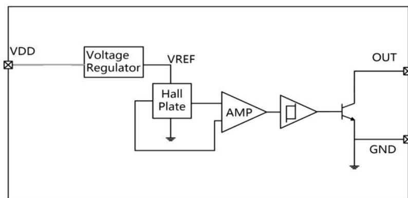
HXY451 功能框图
