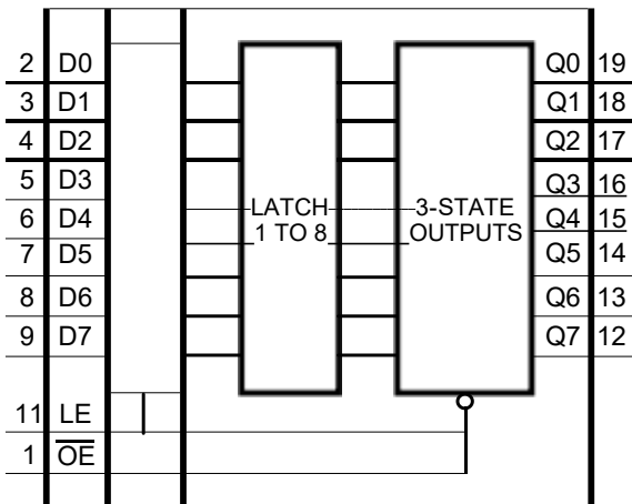
图 3 功能框图
