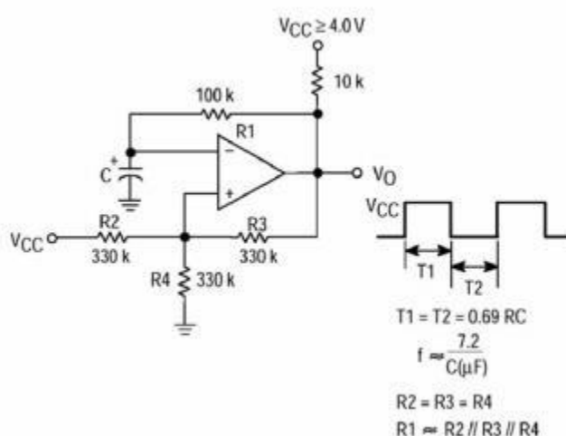
方波振荡器
