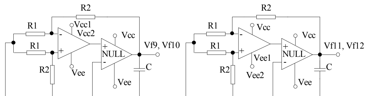
PSRR (+) = 20\log \left| (Vcc1-Vcc2) (1+R2/R1) / (Vf9-Vf10) \right| 电源纹波抑制比 PSRR 测试图
