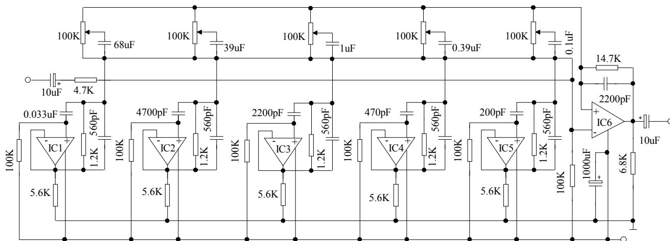
LM324N/NOPB 用于五频率音调控制电路
