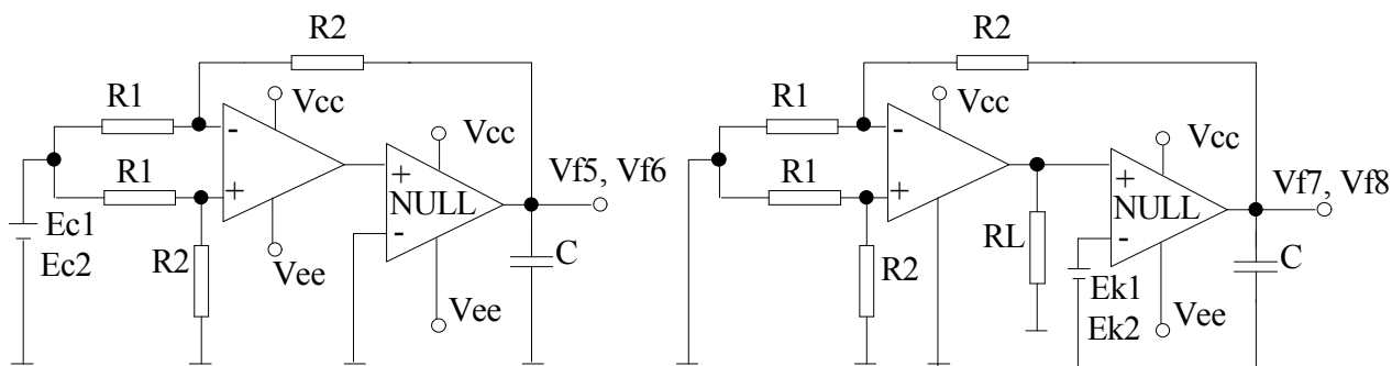
CMR=20\log \left| (Ec1-Ec2) (1+R2/R1) / (Vf5-Vf6) \right| 共模抑制比 CMR 及共模输入电压范围 V_{ICM} 测试图
