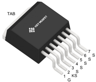
TO-263-7
