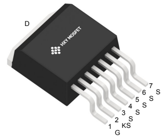
TO-263-7L
