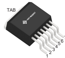
TO-263-7L (TO-263-7-13)
