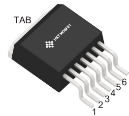
TO-263-7L (TO-263-7)
