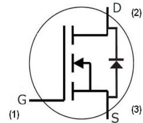
TO-247 (TO-247-3-41)
