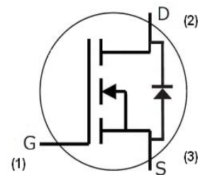
TO-247 (TO-247-3-41)
