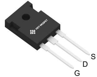
TO-247 (TO-247-3-41)
