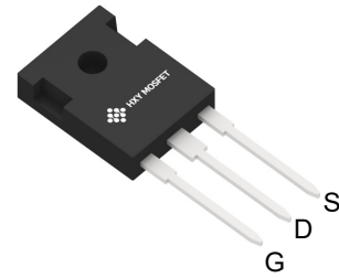
TO-247 (TO-247-3-41)
