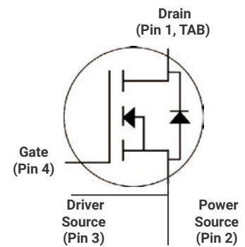
TO-247-4L
