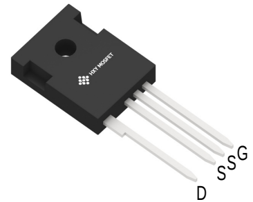
TO-247-4L
