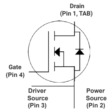
TO-247-4L (TO-247-4)
