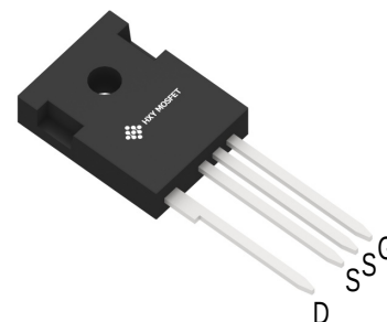
TO-247-4L
