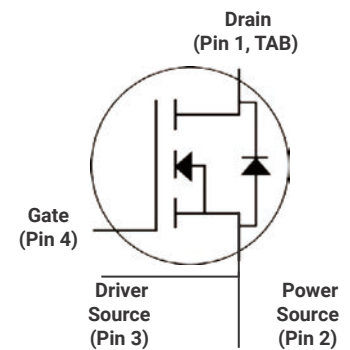
TO-247-4L (TO-247-4)
