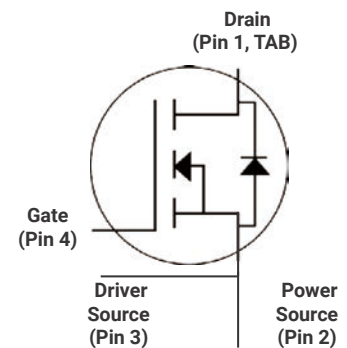
TO-247-4L (TO-247-4)
