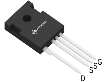
TO-247-4L
