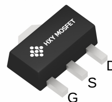
SOT-89 (SC-62)
