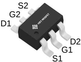
SOT-363
