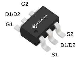
SOT-23-6L
