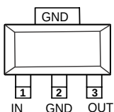
SOT-223
