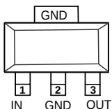
SOT-223
