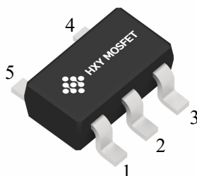
SOT-23-5L (TSOT-23-5)
