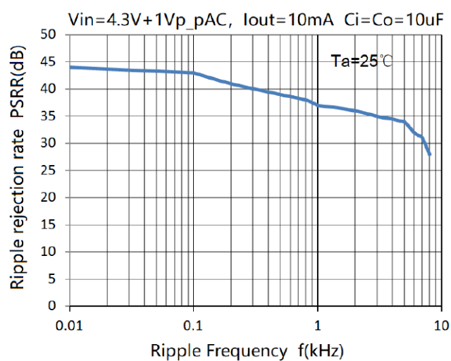
纹波抑制
