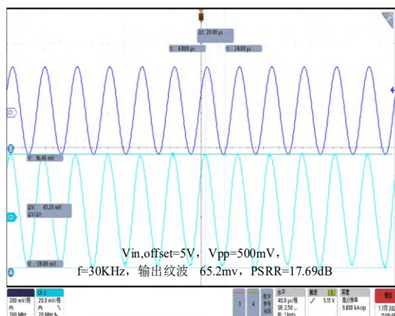
图6 纹波抑制比 (f=30Hz)
