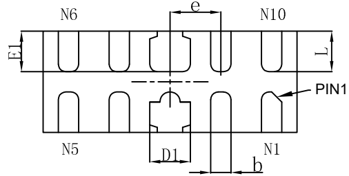
Bottom Vlew
