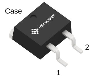
TO-263N
