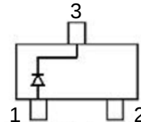
BAT54W
