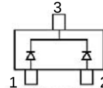
BAT54CW
